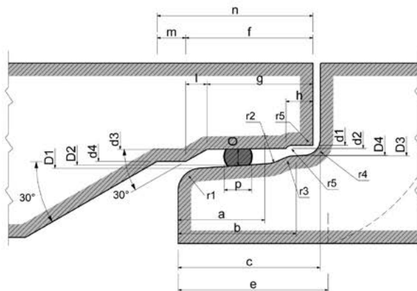
Particolare Giunto
