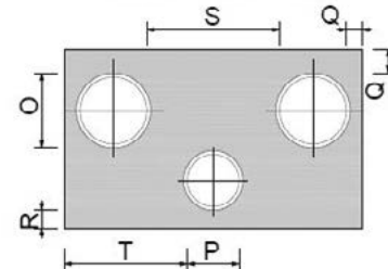
Pianta coperchio
