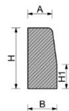
Sezione cordolo vibrocompresso
