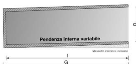
Sezione laterale loculo modulare
