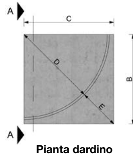
Pianta dardino
