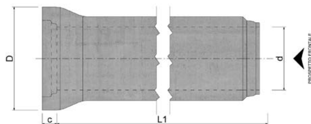
Pianta
