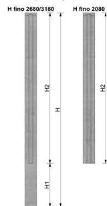
Prospetto pilastrini
