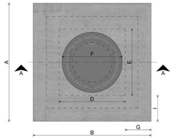
Pianta
