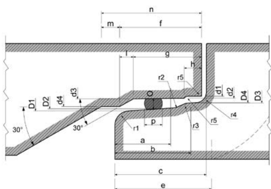
Particolare Giunto
