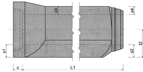
Prospetto laterale
